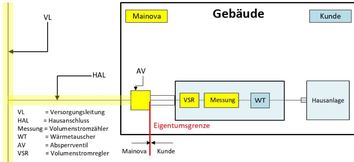
Abbildung 4-1: Eigentumsverhältnisse/Anschlusskizze einer Anlage mit einer Anschlussleistung unter 40 kW
